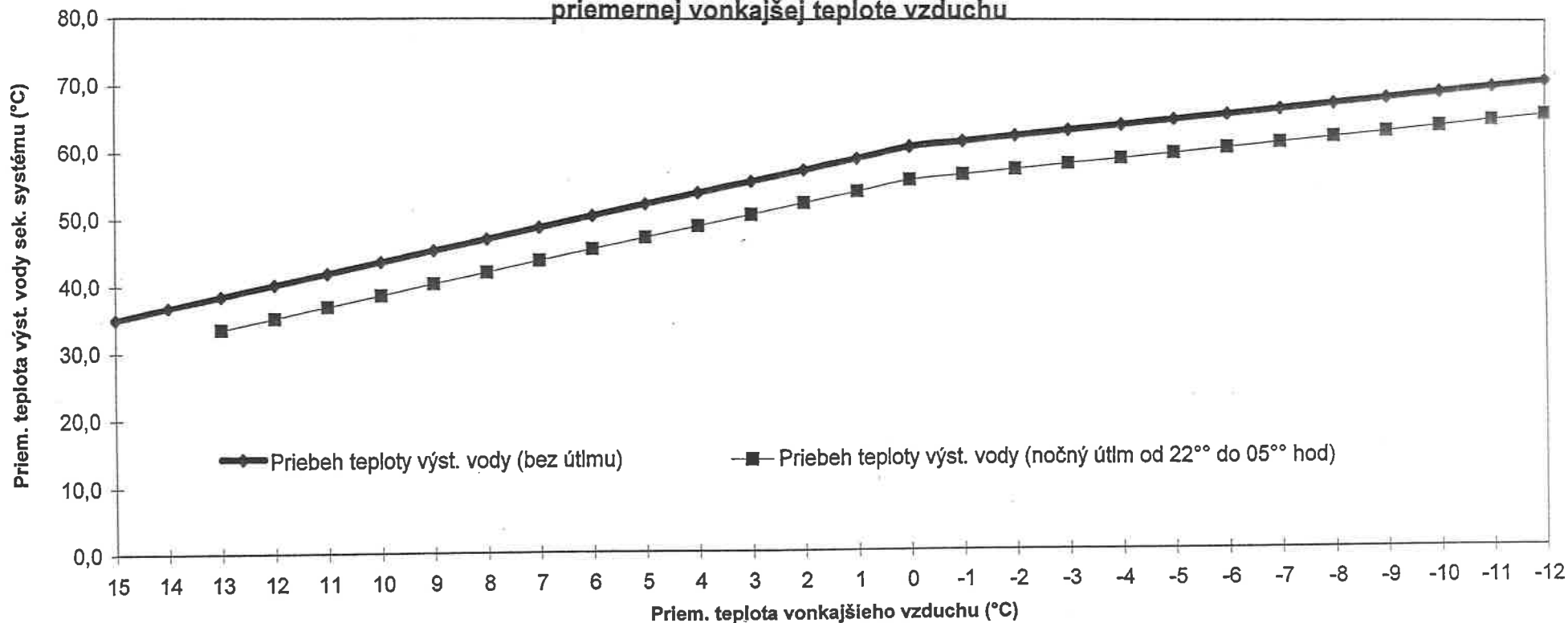
Diagram závislosti priemernej teploty výstupnej obehovej vody sekundárneho systému ÚK na priemernej vonkajšej teplote vzduchu
