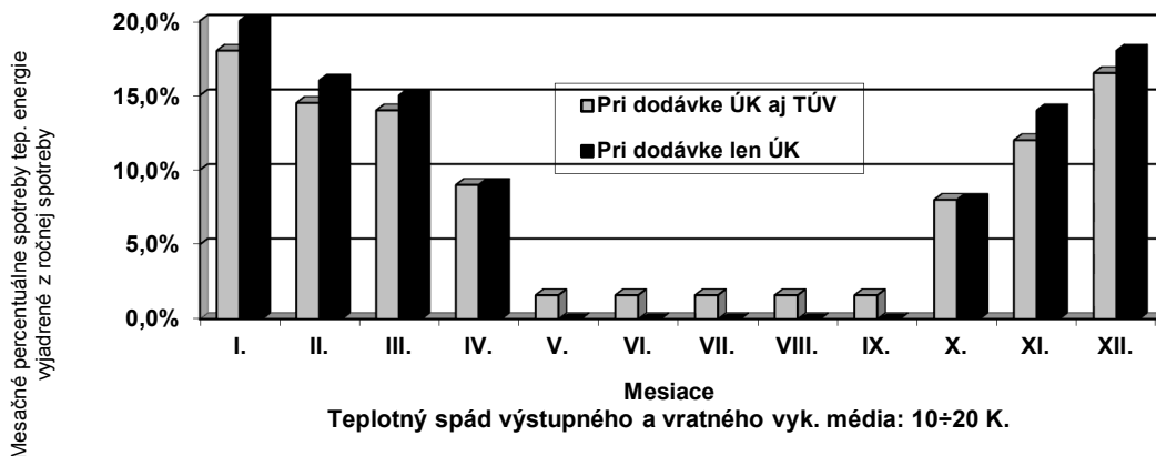
Predpokladaný odberový diagram tepelnej energie
